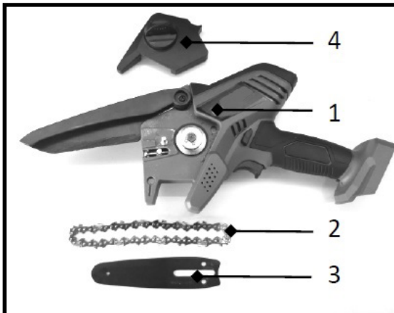
1. Píla 2. Reťaz 3. Vodiaca lišta 4. Kryt pastorka
